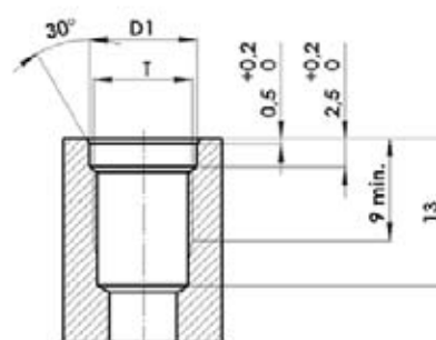
Einschraubloch Form A
