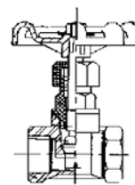
AV-G-NPT 15.07
