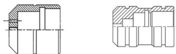
Staubkappe/Stecker 19.07
